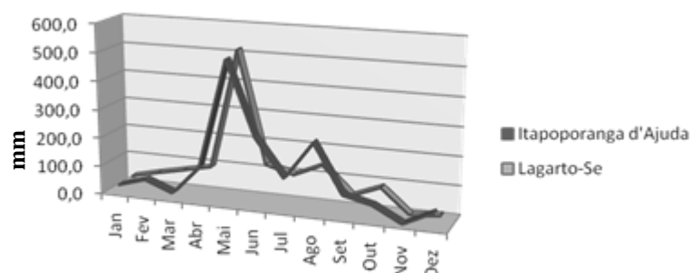
Figura 2: Dados pluviométricos mensal do ano de 2009 dos municípios de Itaporanga d'Ajuda-Se e Lagarto/SE.
